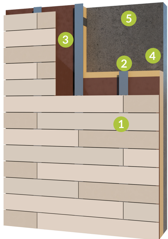
geklebte Montage
