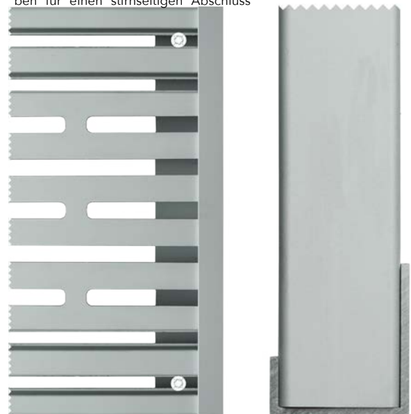
Eck- & Stirnblende B inkl. Systemschrauben für einen stirnseitigen Abschluss
