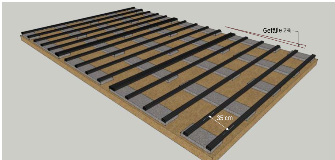
Abb. 2: Befestigung eines Dielenstoßes in der Fläche
